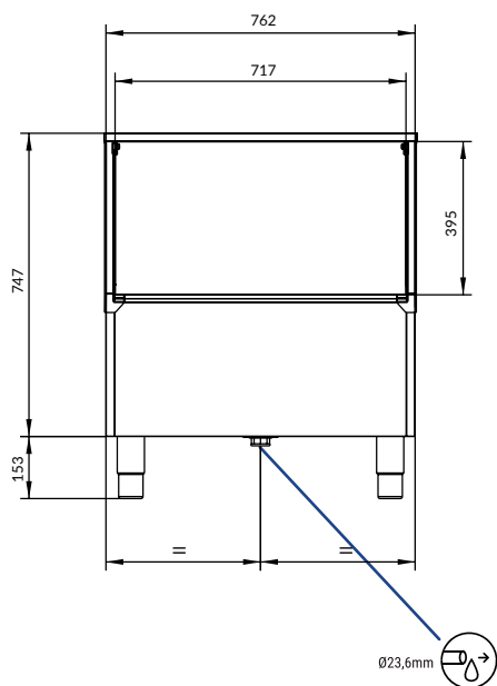
RIGHT SIDE VIEW VISTA LATERAL DERECHA
