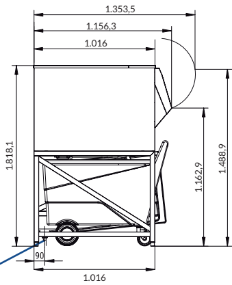
RIGHT SIDE VIEW VISTA LATERAL DERECHA
